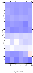
n\_columns
